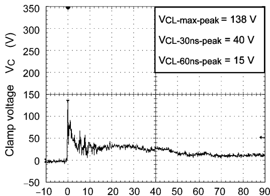
Fig. 10.3 +15 kV
