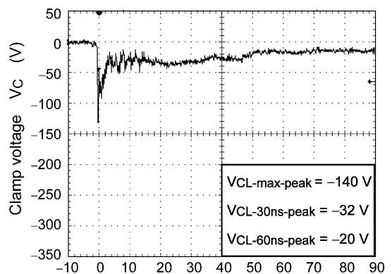
Fig. 10.4 -15 kV
