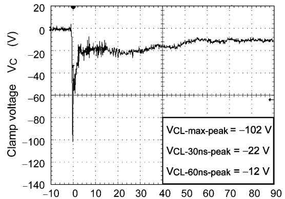
Fig. 10.2 -8 kV
