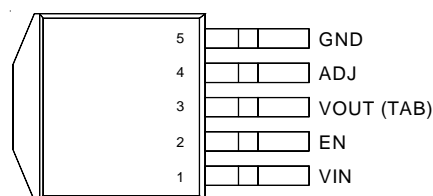
TO-263S-5
